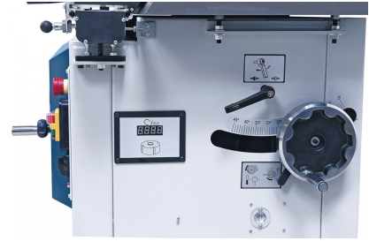
Elektronische Anzeige der eingestellten Fräsgeschwindigkeit.
