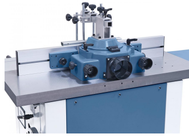
Die Aluminium-Anschlagschienen können schnell und einfach auf das jeweilige Fräs Werkzeug eingestellt werden und sind zusätzlich mit einer Feineinstellung ausgestattet.
