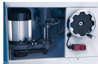
Durch die große Öffnung an der Vorderseite der Maschine kann die Drehzahl schnell und einfach gewechselt werden.
