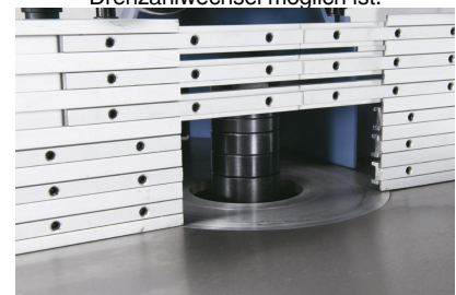
Die Integral-Sicherheitschienen aus eloxiertem Aluminium lassen sich individuell an jede Fräserform anpassen und gewährleisten zusätzlich ein Maximum an Sicherheit.
