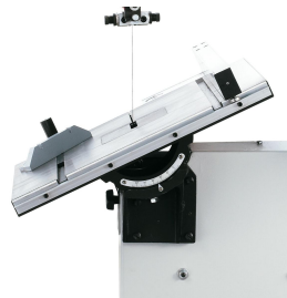
Der Arbeitstisch ist von 0° auf 45° schwenkbar, gewünschte Einstellung mittels Skala ablesbar
