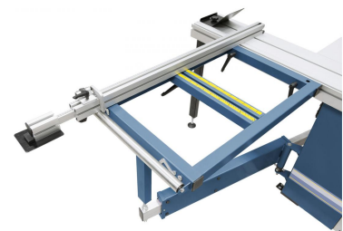
Ausziehbarer Teleskopanschlag (bis 2260 mm) mit feineinstellbarer Anschlagklappe.
