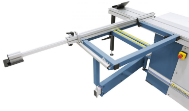
Ausziehbarer Teleskopanschlag (bis 2260 mm) mit feineinstellbarer Anschlagklappe.
