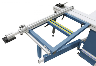
Ausziehbarer Teleskopanschlag (bis 2260 mm) mit feineinstellbarer Anschlagklappe.
