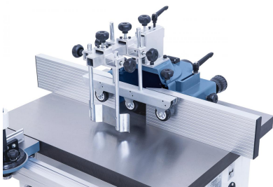
Die Fräseschutzhaube ist mit eloxierten Aluminium-Anschlagsschienen ausgestattet.
