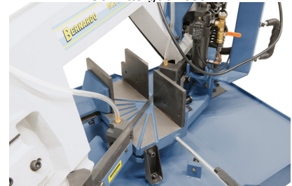
Sägebandführung mit Hartmetall-einsätzen und Spänebürste für optimale Schnittergebnisse.
