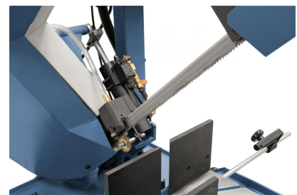
Sägebandführung mit Hartmetall-einsätzen und Spänebürste für optimale Schnittergebnisse.
