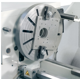
Die serienmäßige Aufspannscheibe diam. 320 mm ermöglicht das Aufspannen von verschieden geformten Werkstücken.
