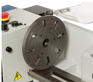
Zum Aufspannen von speziell geformten Werkstücken kann die Maschine mit einer 160 mm Aufspannscheibe ausgerüstet werden.
