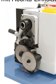
Serienmäßig ausgestattet mit Wechselräder in Metallausführung zum Gewindeschneiden.
