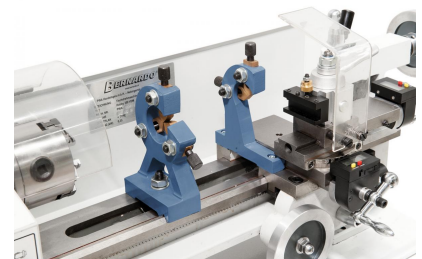
Die Lünetten erleichtern das Bearbeiten von längeren Werkstücken.
