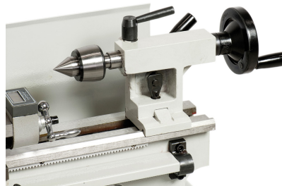
Reitstock mit MK 2 Aufnahme kann zum Kegeldrehen verstellt werden
