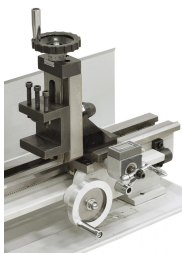
Vertikalfrässupport für zusätzliche Bearbeitungsvorgänge nachrüstbar.
