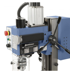
Großdimensionierter Sterngriff für leichte Pinolenzuste beim Bohren, Handrad für Feinzustellung beim Fräsen.
