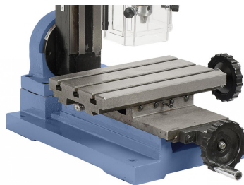
Präzise oberflächenbearbeiteter Kreuztisch mit 3 T-Nuten
