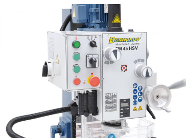
Ergonomisch angebrachte Schalt- elemente an der Vorderseite der Maschine.
