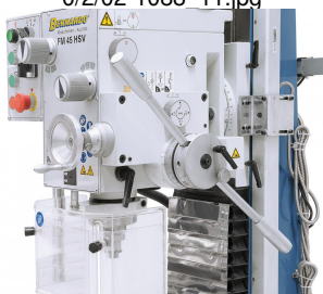
Der Pinolenvorschub kann wahlweise auf 0,10 / 0,18 oder 0,26 mm/U eingestellt werden.
