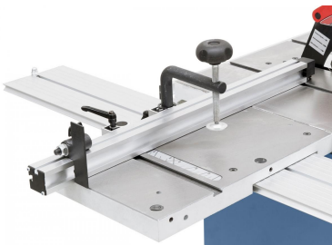
Der Rolltisch aus Grauguss wird plangenaue bearbeitet und geschliffen.
