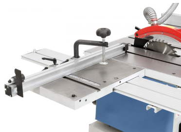
Durch den optionalen Rolltisch mit Aluminiumanschlag und Exzenterstapfen wird der Einsatzbereich zusätzlich erhöht.
