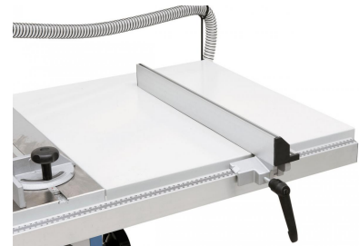
Tischverbreiterung für Schnittbreiten bis 720 mm im Lieferumfang enthalten.
