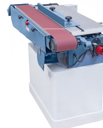
KSM 2740 CN mit horizontal gestelltem Schleifaggregat für erhöhten Einsatzbereich.
