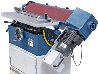
Robuste Schwenkeinrichtung, Schrägstellung des Schleifaggregates von 0° bis 90° möglich.
