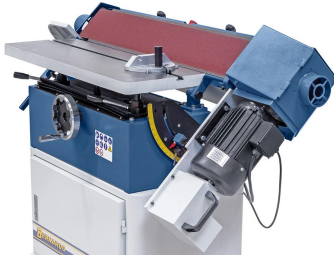
Robuste Schwenkeinrichtung, Schrägstellung des Schleifaggregates von 0° bis 90° möglich.
