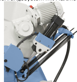
Serienmäßig mit Hydraulik-Absenkzylinder für stufen-loses Absenken des Sägebügels und automatischer Endabschaltung nach Materialdurchschnitt.
