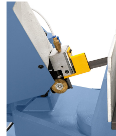
Sägebandführung über kombiniertes Rollen-Backenführungssystem mit Hartmetalleinsätzen
