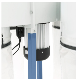
Leistungstarker Motor mit Stahllüfterrad
