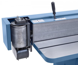
Oszillierendes Schleifaggregat mit 10 mm Hub.
