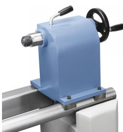
Der Reitstock wird mittels Einhebelklemmung schnell und einfach am Maschinenbett fixiert.
