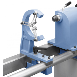
Feststehende Lünette für Wellendurchmesser bis max. 90 mm im Lieferumfang enthalten.
