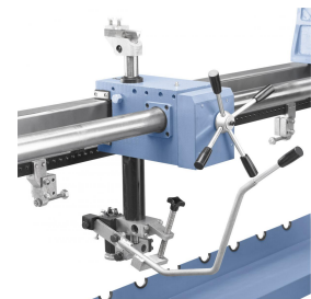
Serienmäßig mit angebaute Kopiervorrichtung, kopieren vom Original oder nach Schablone möglich.
