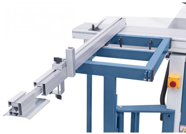
Ausziehbarer Teleskopanschlag, am Auslegertisch vorne und hinten montierbar.
