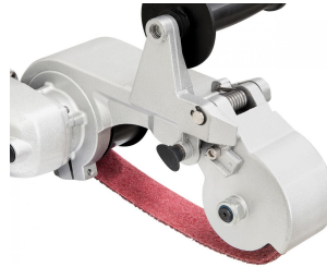
Fixierschraube für schnellen, werkzeuglosen Bandwechsel.
