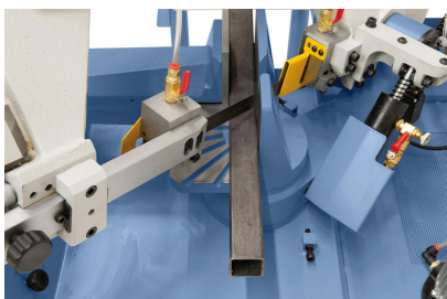
Serienmäßig mit Hydraulikzylinder für stufenloses Absenken des Sägebügels
