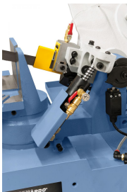
Serienmäßig mit Hydraulikzylinder für stufenloses Absenken des Sägebügels
