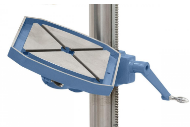
Der Arbeitstisch ist um 360° drehbar, ideal zum Koordinatenbohren.
