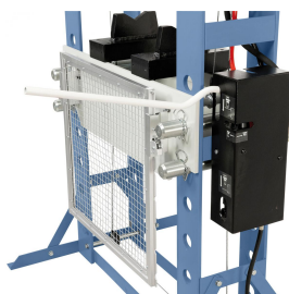
Der Kolbenhub erfolgt wahlweise mittels Handhebel (2 Stufen) oder pneumatisch mittels Fußpedal
