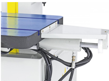
Hydraulikzylinder für Tischvorschub
