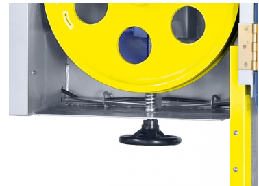
Die Einstellung der Blattspannung erfolgt mittels Handrad.
