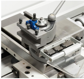
Zum rationellen Arbeiten kann die Maschine mit einem Schnellwechselstahlhalter ausgerüstet werden
