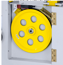
Die dynamisch ausgewuchteten Antriebsräder aus Grauguss sorgen für einen ruhigen Lauf der Maschine.
