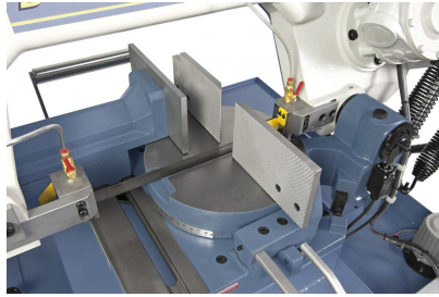
Der Sägeschlitz im Drehteller bewegt sich gleichzeitig mit dem Sägebügel.
