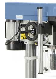
Seitlich positioniertes Handrad zur Einstellung der gewünschten Drehzahl
