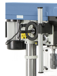
Seitlich positioniertes Handrad zur Einstellung der gewünschten Drehzahl
