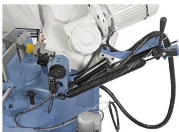
Zugfeder mit Einstellhebel zum Umstellen auf manuellen Betrieb.
