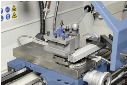
Schnellwechselstahlhalter System Multifix im Lieferumfang enthalten
