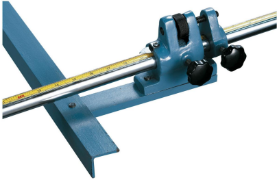
Der Hinteranschlag ist serienmäßig mit einer Feineinstellung ausgestattet
