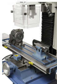
Halb-Universal-Teilkopf BS-0: optimal für die Wellenbearbeitung
