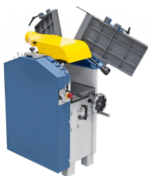
Die hochklappbaren Abrichttische ermöglichen beim Dickenhobeln ein optimales und sicheres Arbeiten, auch bei kurzen
