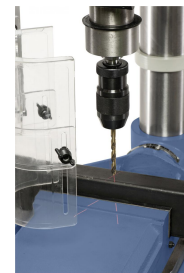
Präzises Arbeiten durch die serienmäßige Kreuzlinien-Lasereinrichtung
