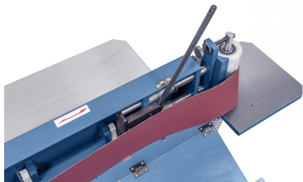
Bedienerfreundliches Wechseln des Schleifbandes durch Schnellspanneinrichtung.
