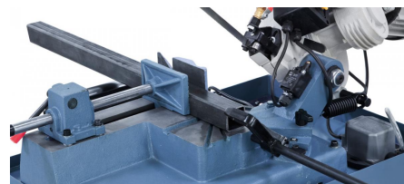
Einfache Verstellung des Schraubstockes mittels Schnellspannhebel
